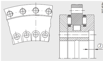
对于 YRT80-TV 和 YRT100 : ② 螺栓沉头孔开口方向 3)
