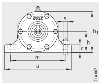
横截面
