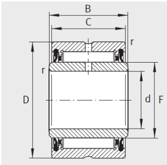
NA4908-2RSR
