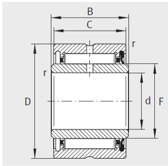
NA49..-RSR
